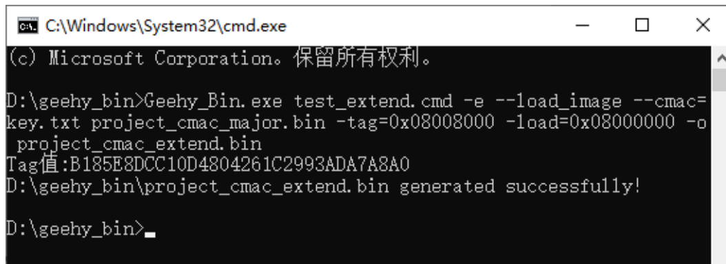
图 4 生成扩展安全启动的 Golden CMAC Tag 值的 bin 文件
